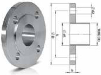
PASLANMAZ PN10-PN16-PN25-PN40 DÜZ FLANŞLAR
