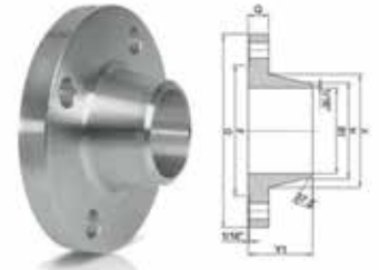
PASLANMAZ 150-300 Lbs KAYNAK BOYUNLU FLANŞ
